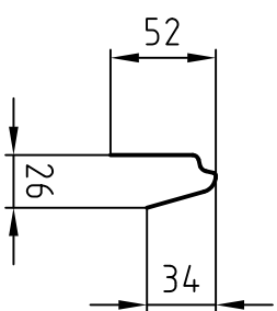
Schnitt A-A
