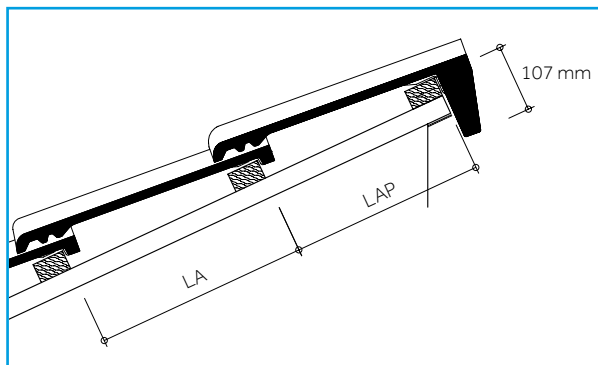
Pultsteine für Tegalit
