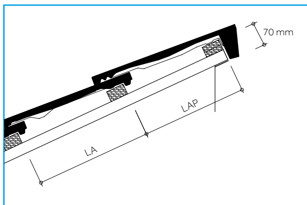
Pultsteine für Tegalit Aerlox
