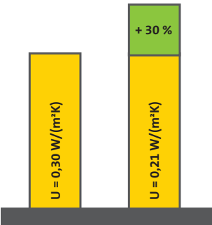
Vergleich Dämmqualität : reine Zwischensparren-Dämmung im Vergleich zur Zwischensparren-Dämmung mit kombinierter Untersparren-Dämmung. 60 mm zusätzliche Untersparren-Dämmung bewirken eine Verbesserung der Dämmleistung des Bauteils Dach um 30%.
