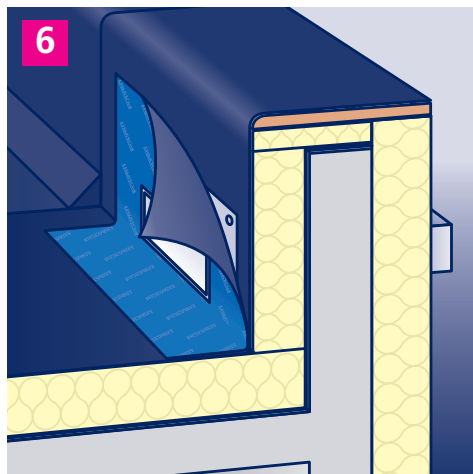
6. An den vorgegebenen Punkten mechanisch fixieren. Ringspalt verschließen und abdichten. Ggf. Wandscheibe für Speier (nicht inkl.) montieren.
