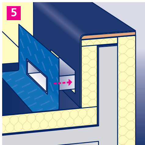
5. Den Speier durch die Dampfsperplatte und die Attika führen.
