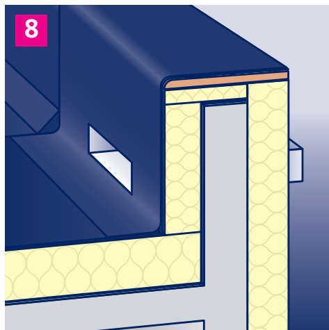
8. Oberlage aufschweißen oder -kleben. Ggf. Speier-Kiesfang montieren.
