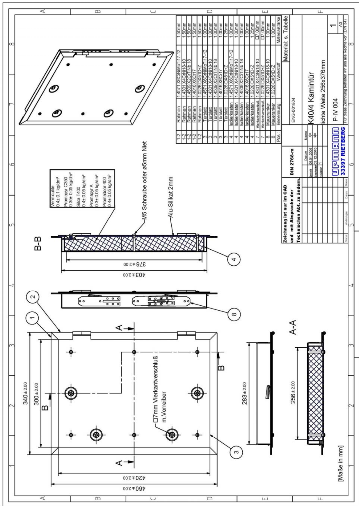
Schornsteinreinigungsverschluss "K40" Rahmen und Tür aus nichtrostendem oder verzinktem Stahlblech, lichte Reinigungsöffnung 256 mm x 376 mm
