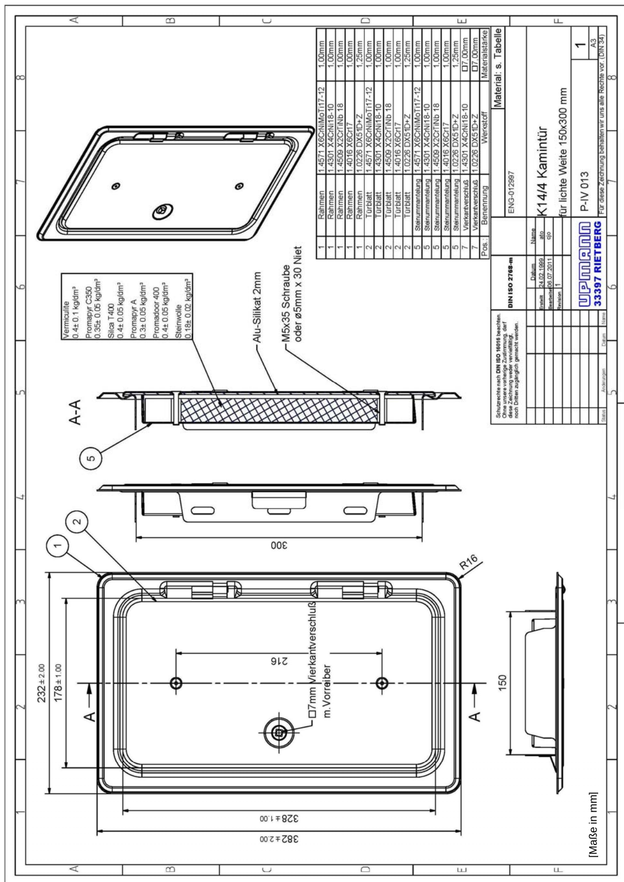
Schornsteinreinigungsverschluss "K14" Rahmen und Tür aus nichtrostendem oder verzinktem Stahlblech, lichte Reinigungsöffnung 150 mm x 300 mm
