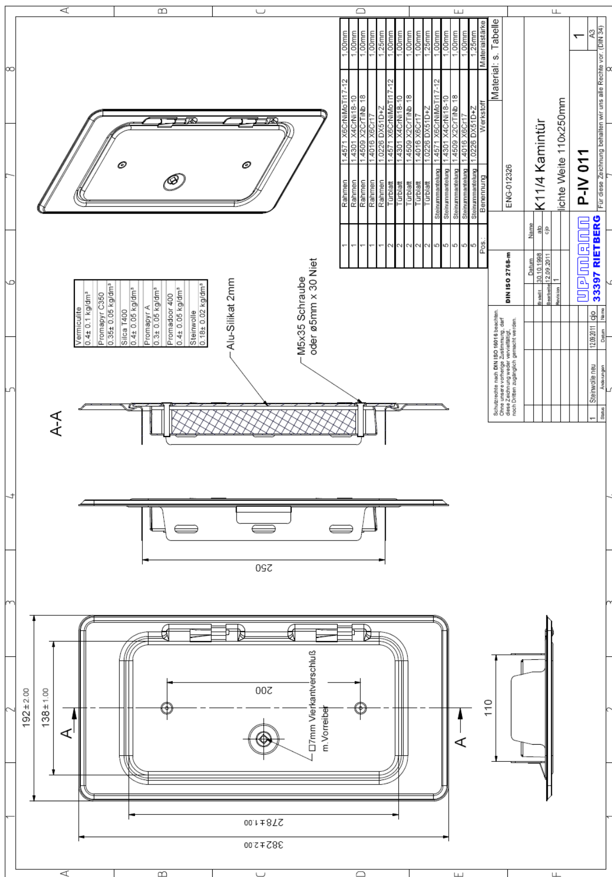
Schornsteinreinigungsverschluss "K11" Rahmen und Tür aus nichtrostendem oder verzinktem Stahlblech, lichte Reinigungsöffnung 110 mm x 250 mm
