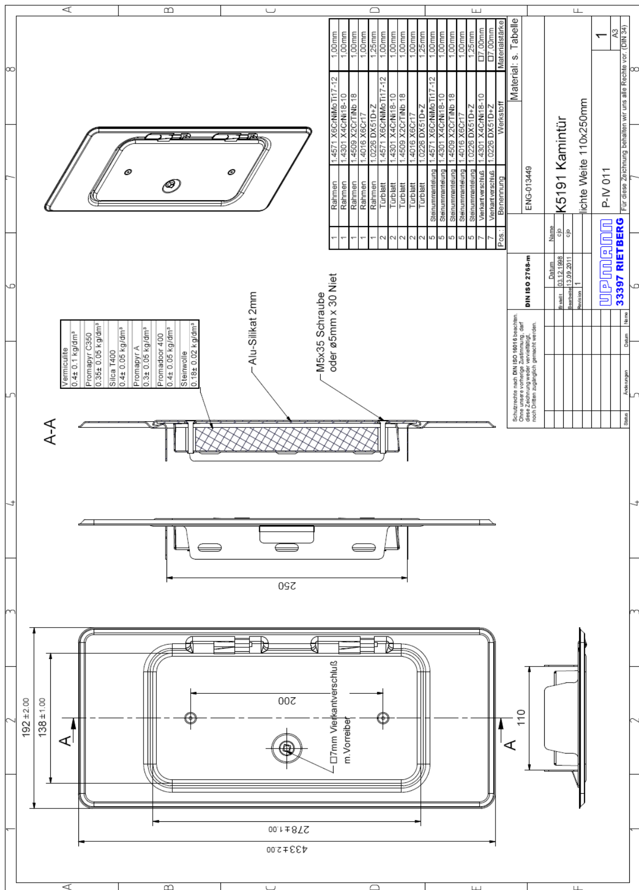
Schornsteinreinigungsverschluß "K5191" Rahmen und Tür aus nichtrostendem oder verzinktem Stahlblech, lichte Reinigungsöffnung 110 mm x 250 mm
