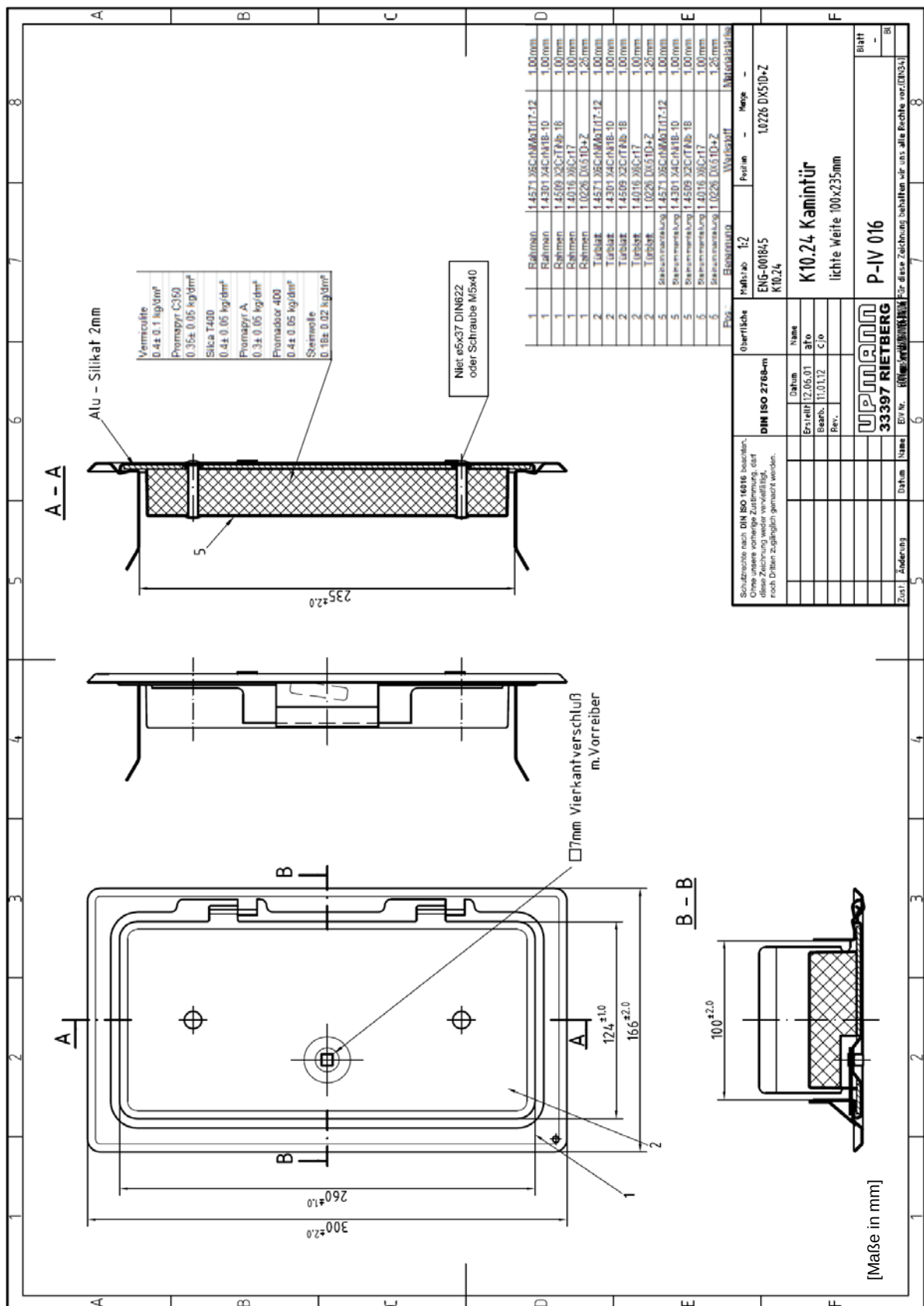
Schornsteinreinigungsverschluss "K10.24" Rahmen und Tür aus nichtrostendem oder verzinktem Stahlblech, lichte Reinigungsöffnung 100 mm x 235 mm
