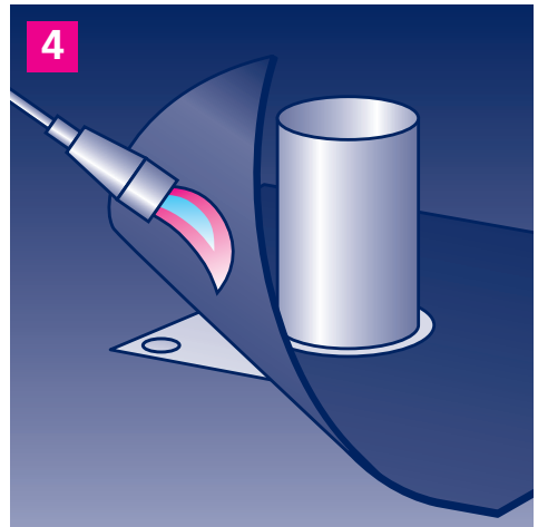
4. Anschlussstück des Flachdachdunstrohrs durch Verschweißen oder Verkleben mit der Abdichtung verbinden. Ggf. Haube oder Zugverstärker (siehe Rückseite) aufstecken.
