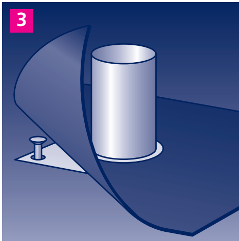
3. Flachdachdunstrohr mit geeigneten Befestigungsmitteln mechanisch mit dem Untergrund verbinden.
