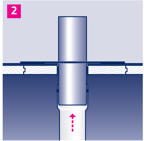
2. Flachdachdunstrohr ausrichten und ein Entlüftungsrohr anschließen.
