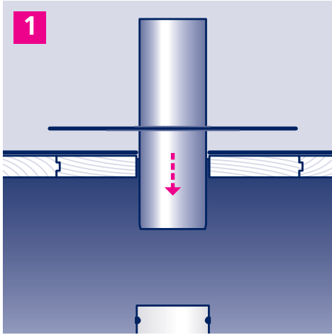
1. Flachdachdunstrohr durch die vorbereitete Öffnung im Dach stecken.
