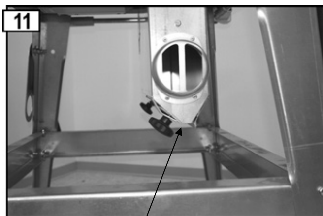
Fessura espulsione trucioli aperta (funzionamento senza dispositivo per l'aspirazione dei trucioli)
