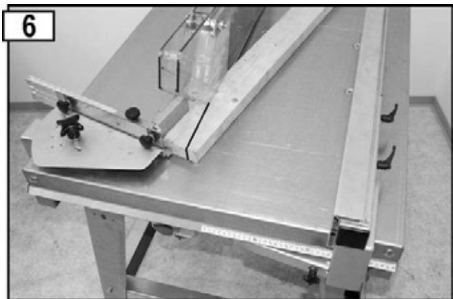
Couper des coins à l'aide de la butée à coins
