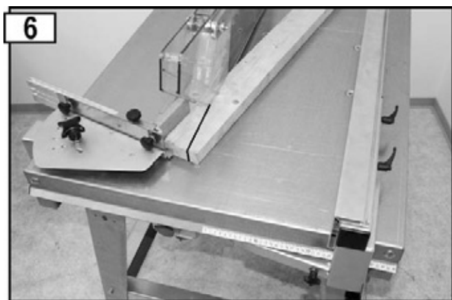
Klíňové řezy s klínovým dorazem
