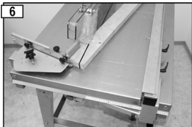
Taglio a cuneo con l'apposita guida di arresto
