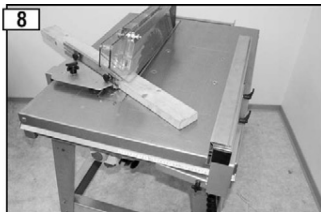
Utilizarea opritorului transversal mobil
