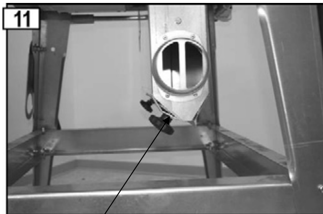
Spanauswurfschlitz offen (Betrieb ohne Späneabsaugvorrichtung)
