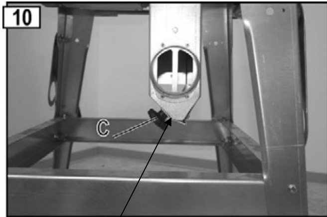
Spanauswurfschlitz geschlossen (Betrieb mit Späneabsaugvorrichtung)
