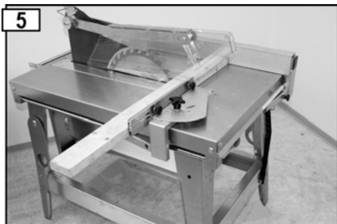
Guida parallela come guida per tagli trasversali
