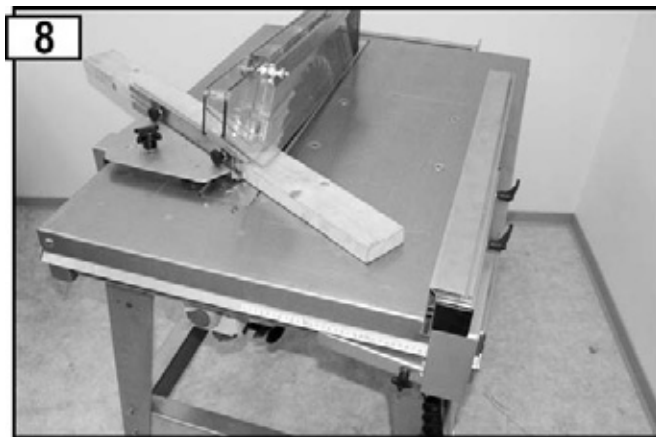
Utilisation de la butée transversale amovible
