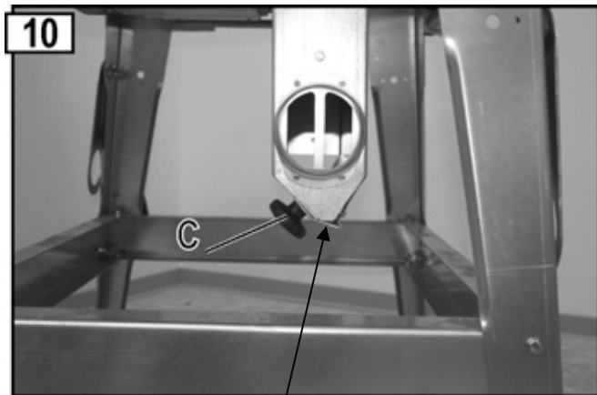
Fessura espulsione trucioli chiusa (funzionamento con dispositivo per l'aspirazione dei trucioli)
