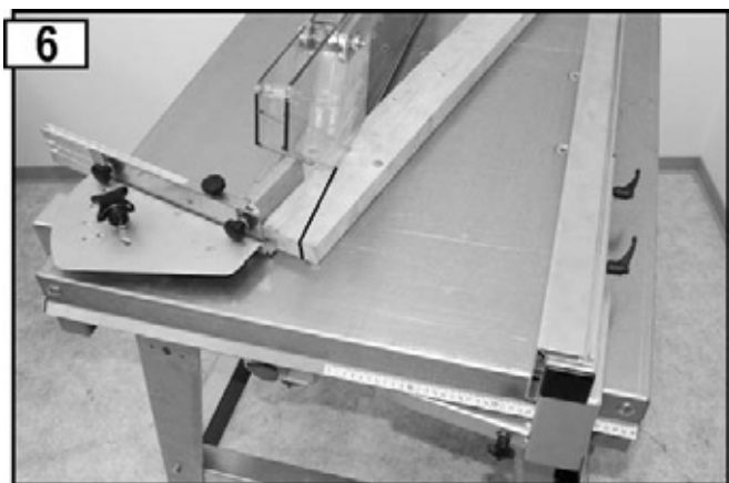
Tăierea cu opritorul pentru tăietură în formă de pană
