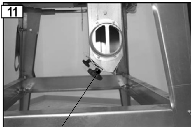
Szczelina do wyrzucania wiórów (praca z wyciągiem)
